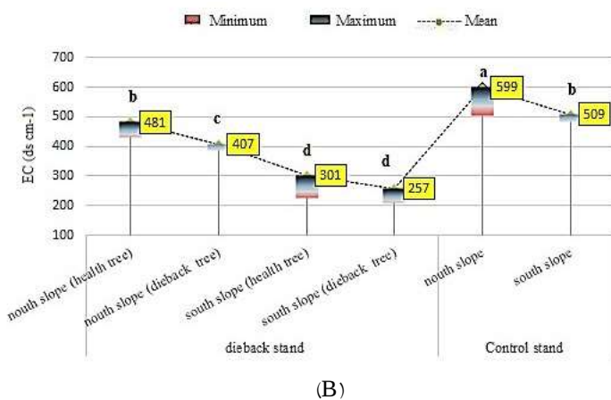
شکل ۳- میانگین pH (A) و هدایت الکتریکی (B) در قطعات نمونه گاران و دوله‌ناو
