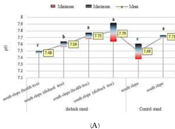
شکل ۳- میانگین pH (A) و هدایت الکتریکی (B) در قطعات نمونه گاران و دوله‌ناو
