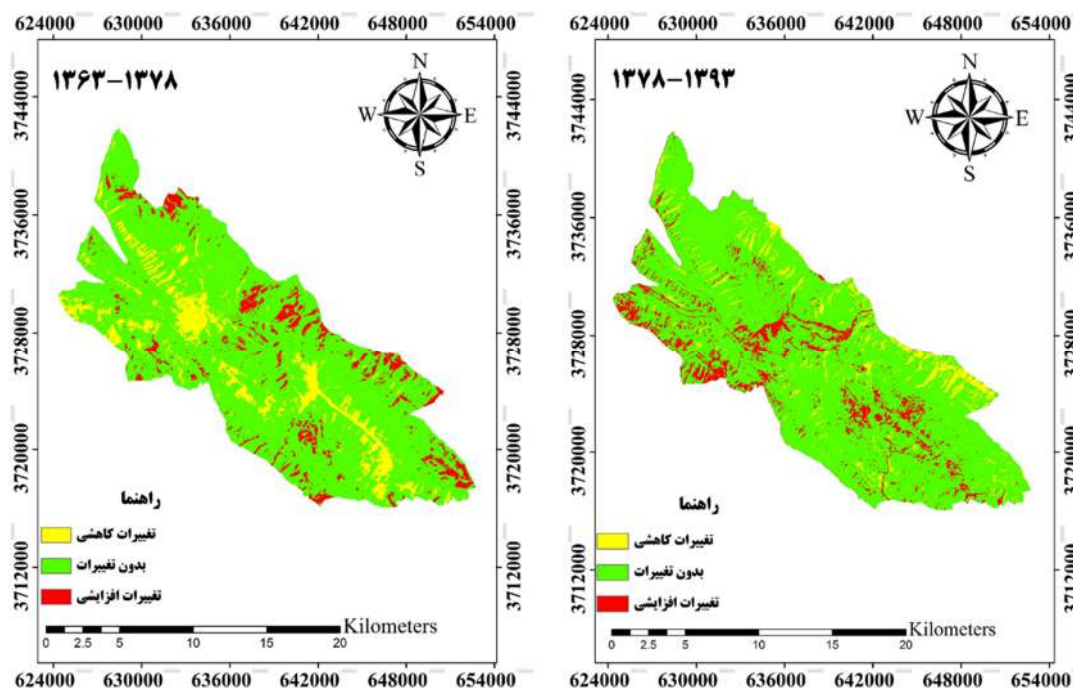
شکل ۶- نقشه تفاضل تجزیه مؤلفه‌های اصلی (PCA) حاصل از باند سوم و آستانه دوم در دوره‌های زمانی مطالعه شده (۱۳۷۸-۱۳۹۳ و ۱۳۶۳-۱۳۷۸)
