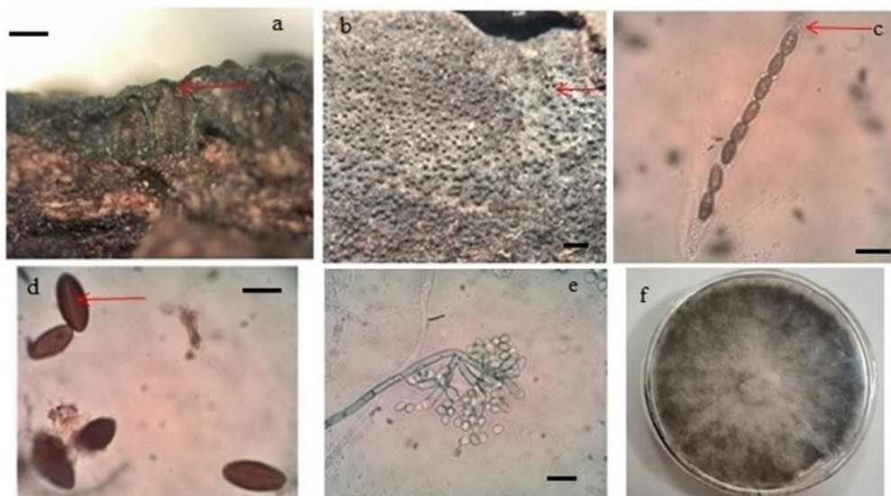
شکل ۱- مرفولوژی قارچ Biscogniauxia mediterranea -a نمای جانبی آسکوکارپ و دهانه آن (Bar=200µm) -b نمای سطحی استروما و دهانه برجسته آسکوکارپ (Bar=500µm) -c اسپورهای ردیفی داخل آسک -d اسپور به همراه خط تندش (Bar=20µm) -e نمای میکروسکوپی قارچ (Bar=10µm) -f منظره رویش ۱۴ روزه در محیط PDA
