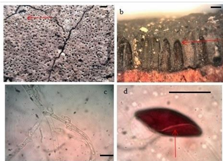
شکل ۲- مرفولوژی قارچ Obolarina persica -a نمای سطحی استروما و دهانه فرورفته پریتیس (Bar=200µm) -b نمای جانبی پریتیس و دهانه آن (Bar=500µm) -c نمای میکروسکوپی قارچ (Bar=20µm) -d اسپور به همراه خط تندش (Bar=20µm)
